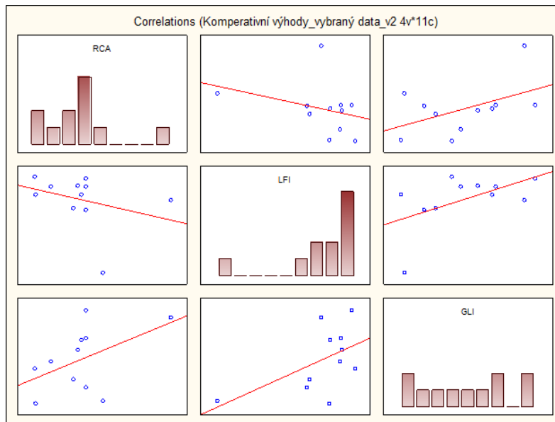
Graf č. 21: Korelace RCA, LFI a GLI v případě cukrovinek za Itálii
