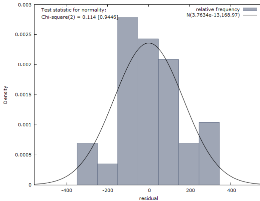
Graf č. 22: Histogram normality reziduí první rovnice
