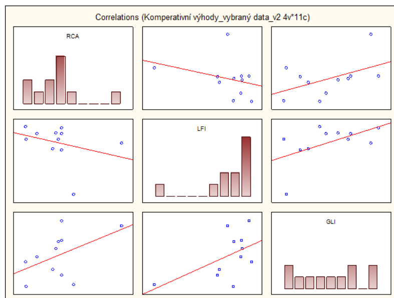
Graf č. 19: Korelace RCA, LFI a GLI v případě cukrové řepy za Itálii
